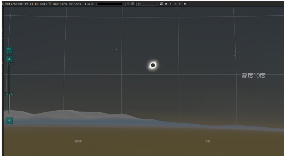
地形のシミュレート (ステラナビゲータ®による) ※参考程度にお考えください。
