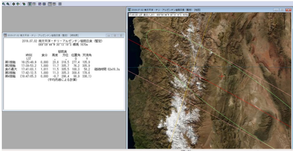
観測場所での日蝕時刻表 (エクリプスナビゲータ®による)
