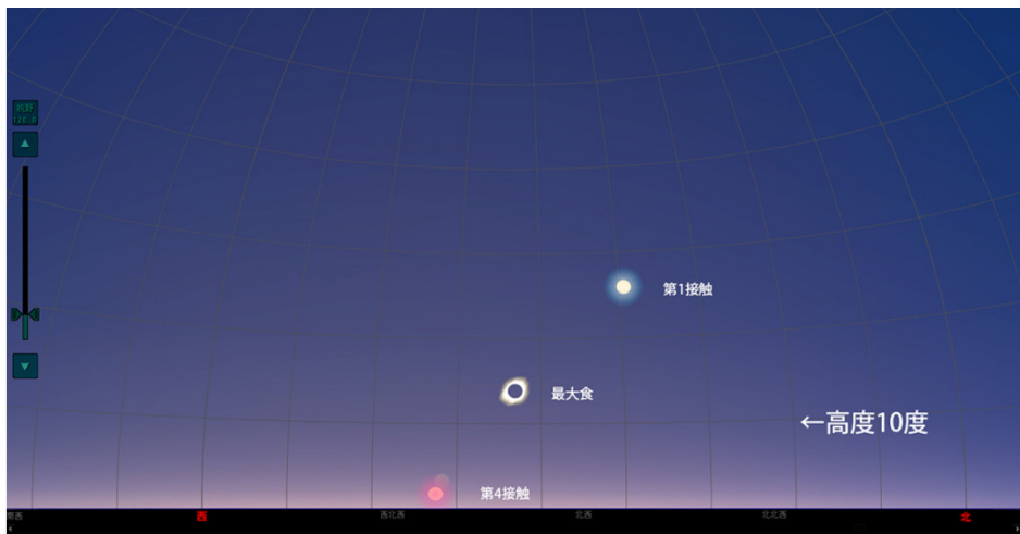
第1接触、最大食、第4接触を合成した予想図（ステラナビゲータ®による）※参考程度にお考えください。
